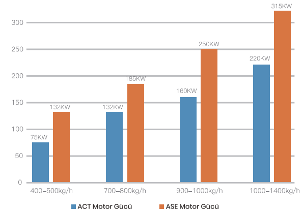
ACT Konik İkiz Vidalı Ekstrüder ile ASE Tek Vidalı Ekstrüder Arasındaki Enerji Tüketimi Karşılaştırma Tablosu
